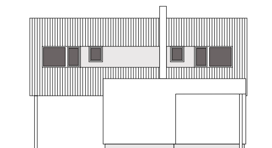
POHLED P3
